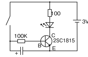
⑪フルカラーLED点灯回路
